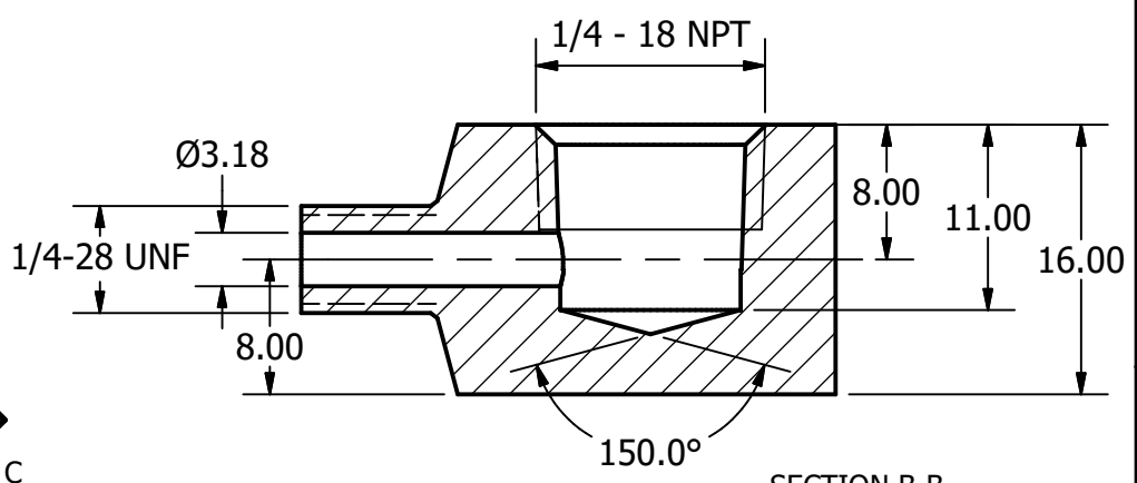
SECTION B-B SCALE 2 : 1
